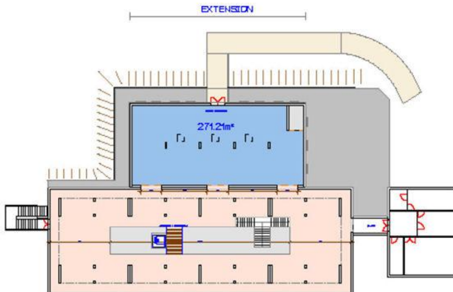
Vue de dessus de tout le premier étage montrant l'extension en bleu et le plan incliné servant d'issue de secours en jaune pâle
